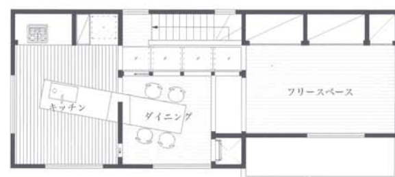
改修2階平面図
