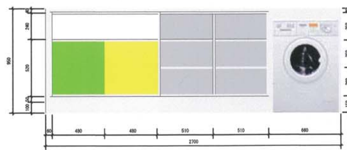
C面 側面図
