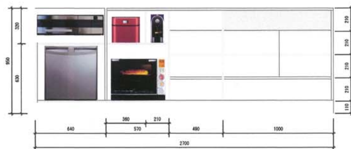
A面 側面図
