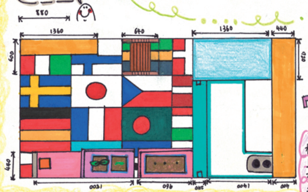
1F平面図 S1:40
