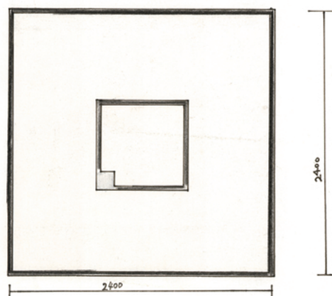
平面図 B1F 1/30
