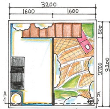
平面図 S=1:50
