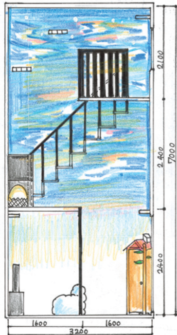
A-A'断面図 S=1:50
