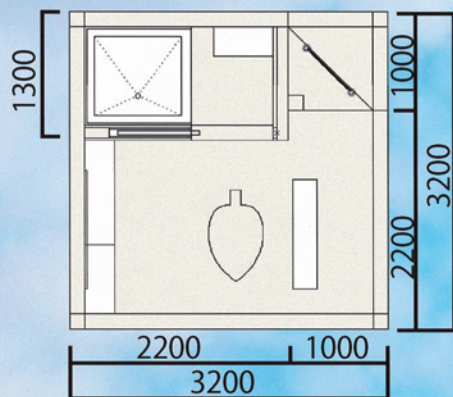
一階平面図 1/50
