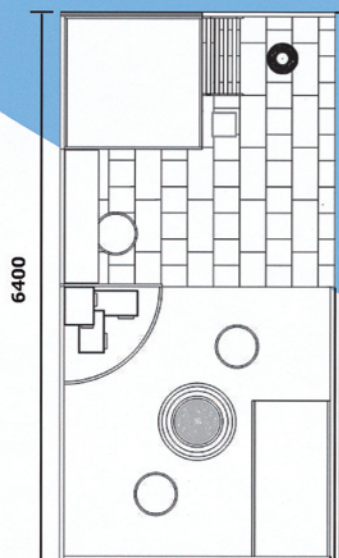
平面図 1:50
