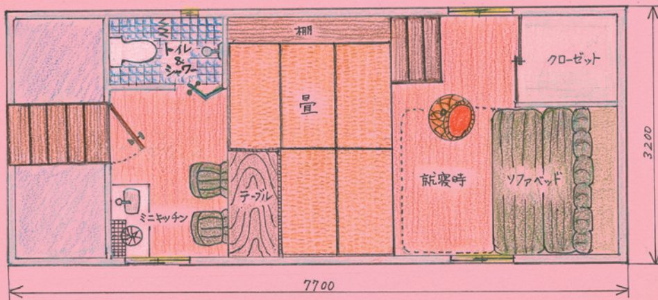
平面図 1/40
