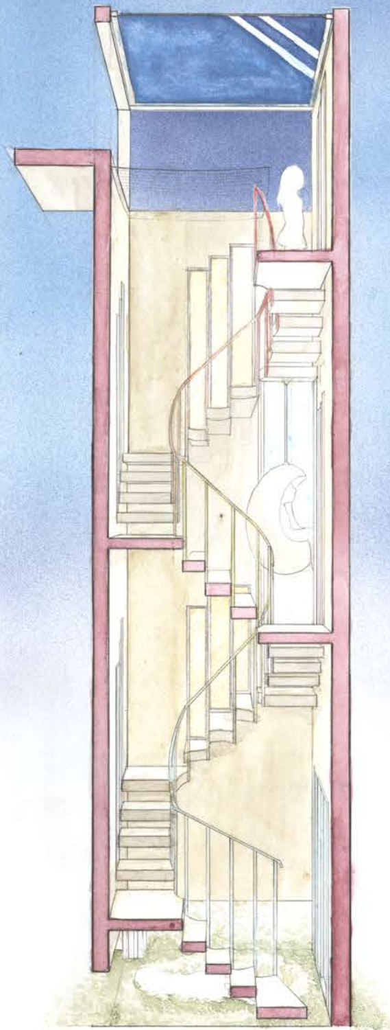
断面パース Scale 1:30
