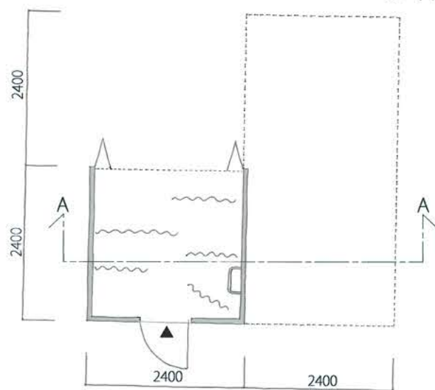
2F 平面図
