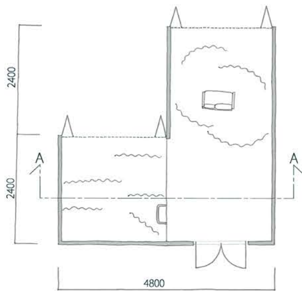
2F 平面図
