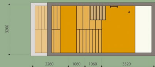
平面図 1/60
